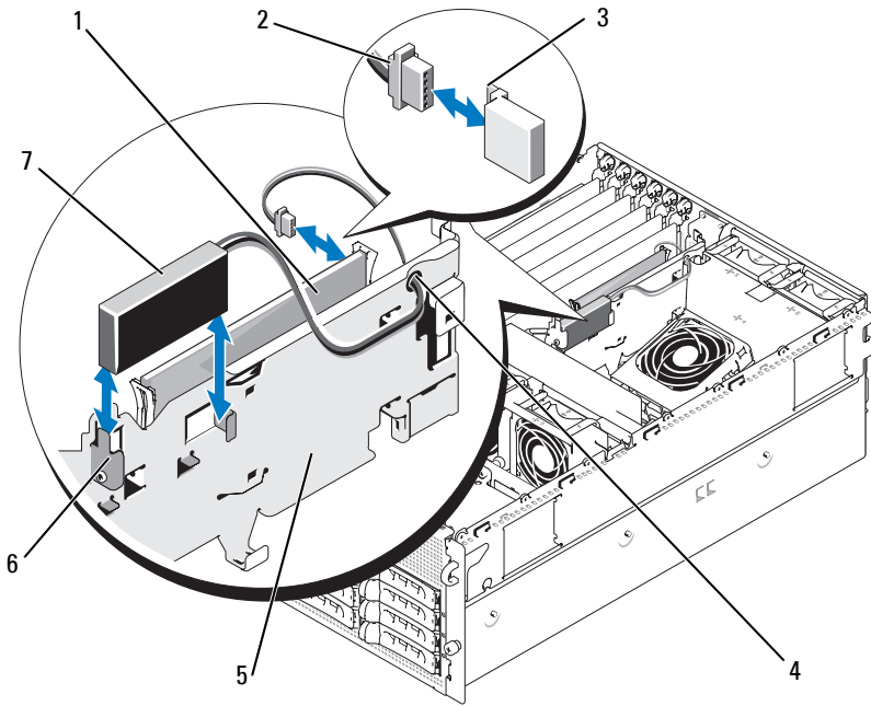
图 3-27. 更换 SAS RAID 控制器子卡电池
