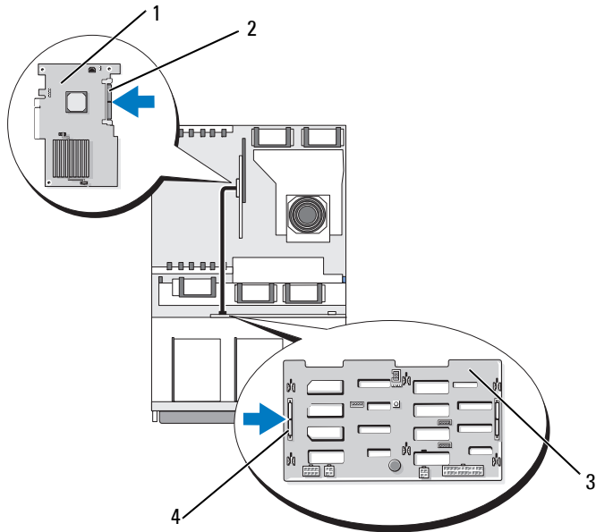
图 3-29. (非 RAID) SAS 控制器的布线
