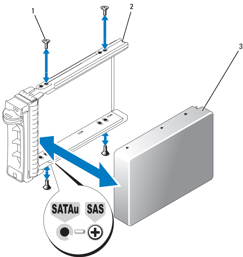
图 3-7. 将 SAS 硬盘驱动器安装到驱动器托盘中
