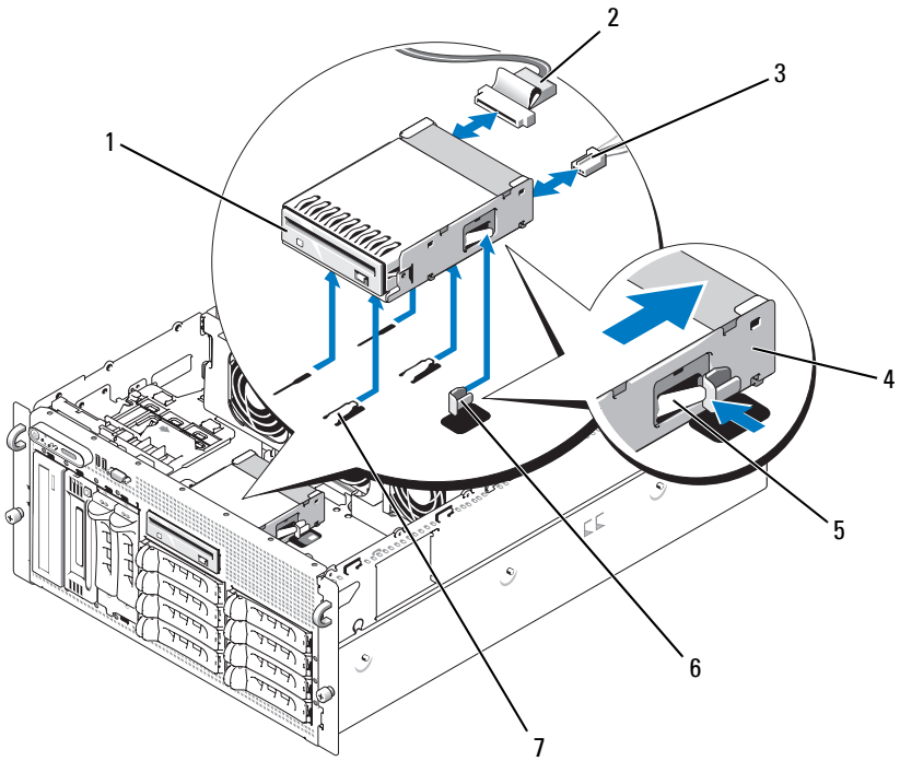
图 3-17. 安装和卸下软盘驱动器
