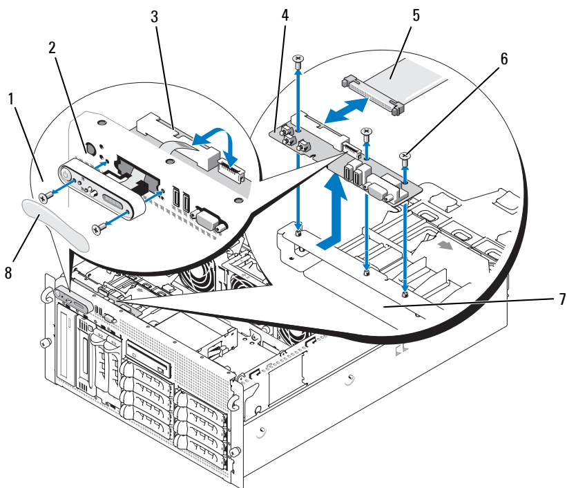
图 3-32. 卸下控制面板部件
