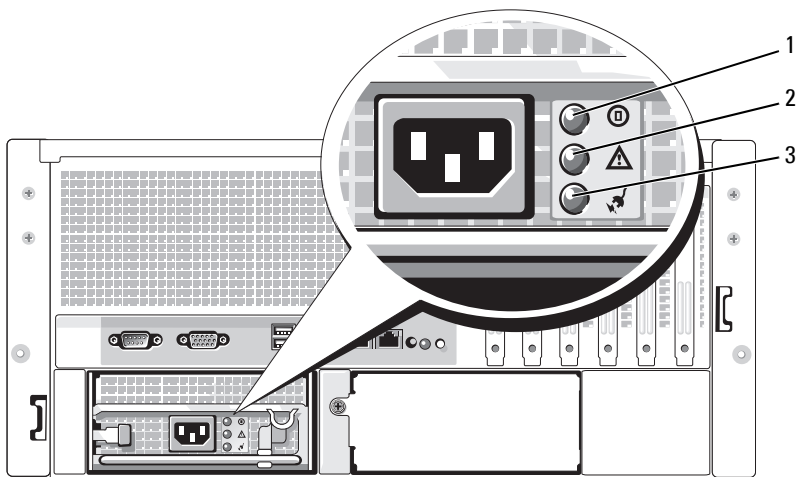
图 1-5. 冗余电源设备指示灯
