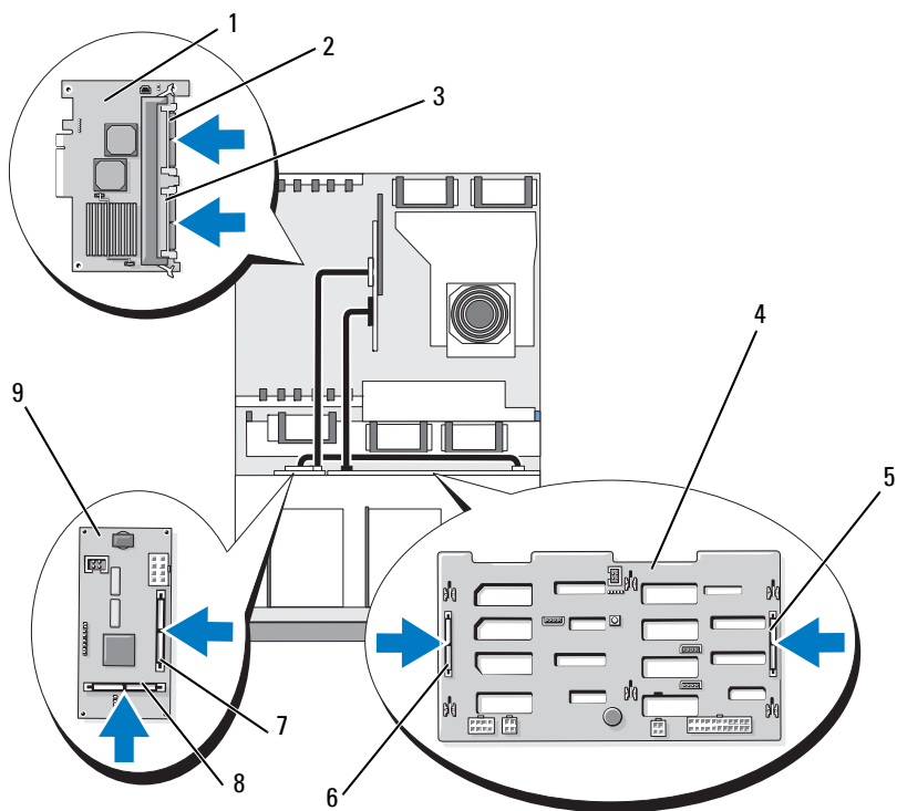
图 3-31. 将 SAS RAID 控制器连接至 1x8 和 1x2 背板
