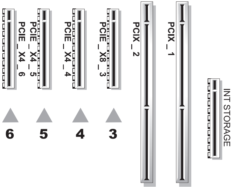
图 3-14. 扩充槽
