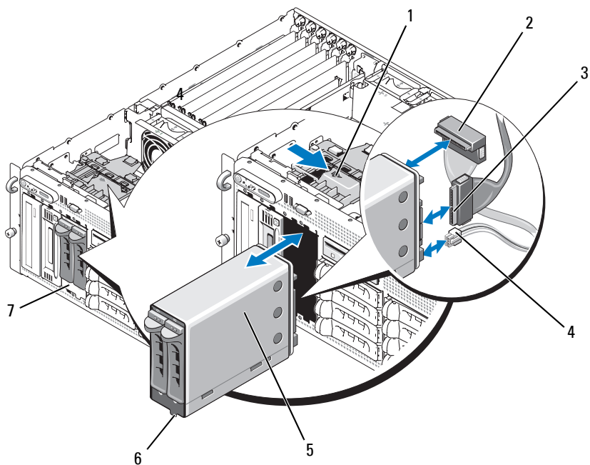
图 3-26. 安装和卸下可更换托架驱动器支架
