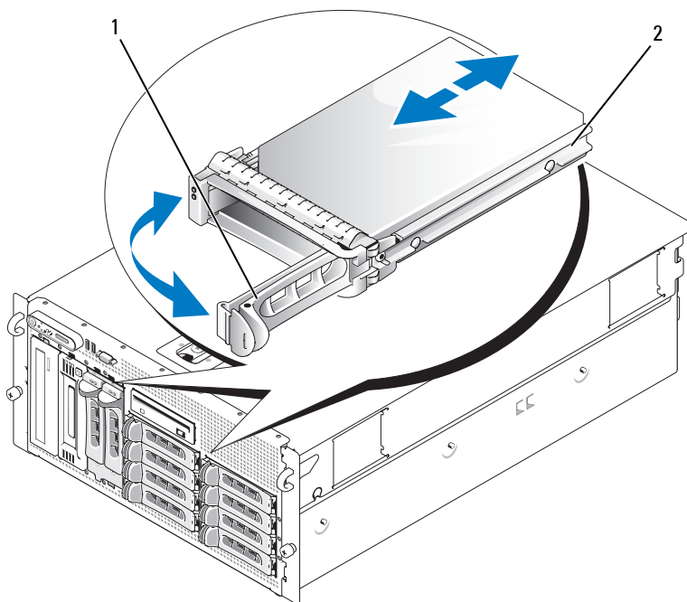
图 3-6. 安装热插拔硬盘驱动器
