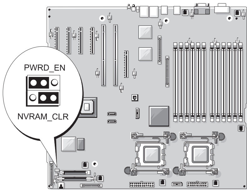
图 6-1. 系统板跳线
