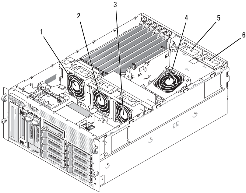
图 3-11. 冷却风扇
