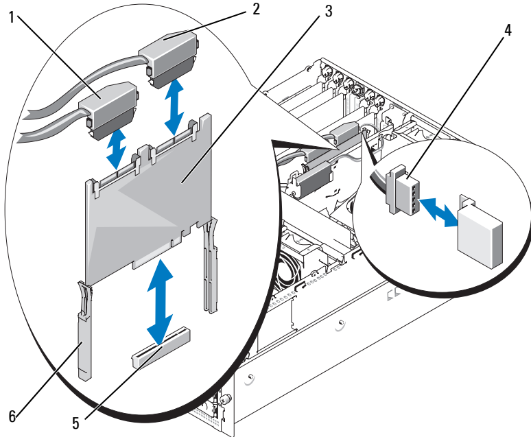
图 3-28. 安装和卸下 SAS 控制器子卡
