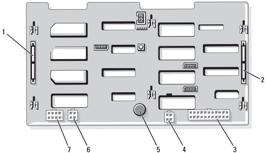
图 6-3. 1x8 SAS 背板连接器
