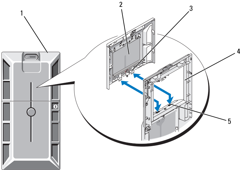
图 3-3. 安装和卸下外围设备托架面板（塔式）
