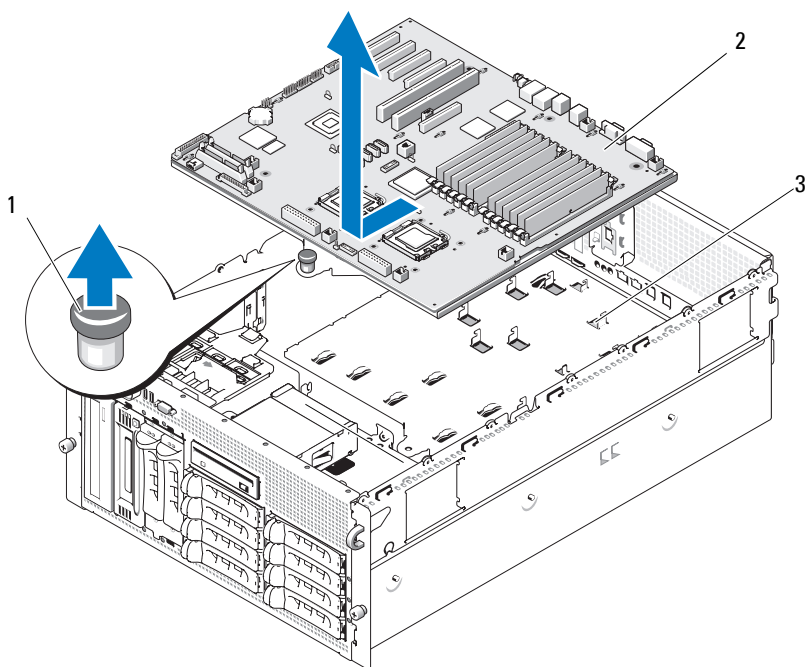
图 3-33. 卸下系统板
