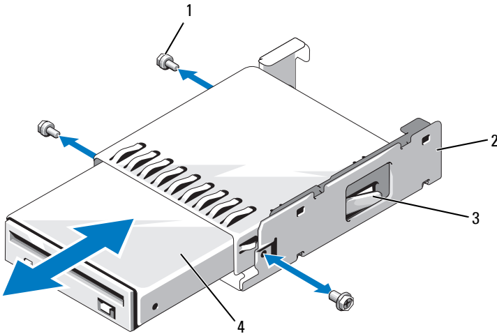
图 3-18. 将软盘驱动器安装到驱动器托盘中
