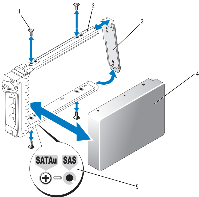
图 3-9. 将 SATA 硬盘驱动器和插入器卡安装到 SATAu 驱动器托盘中
