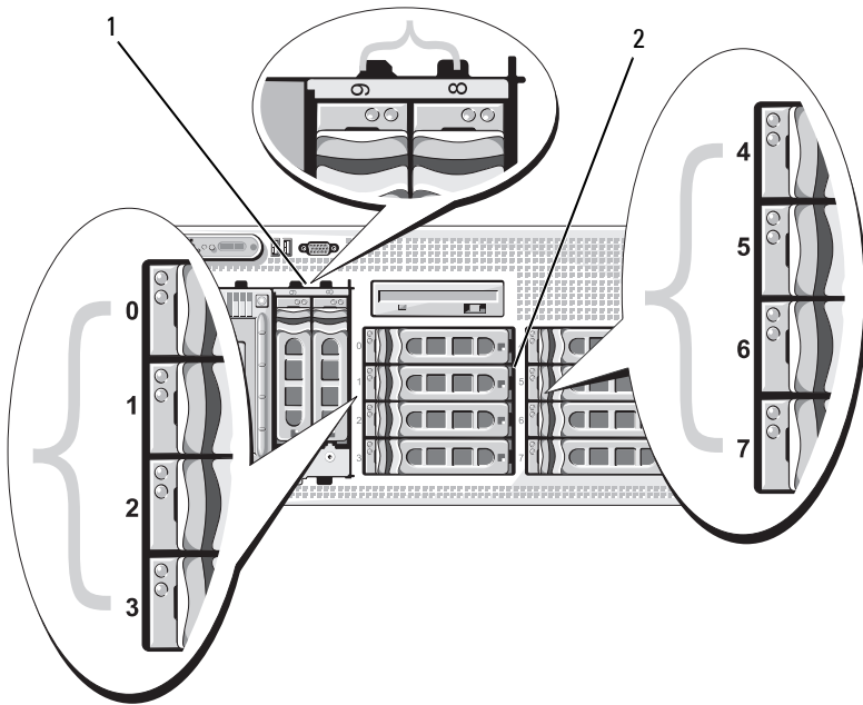
图 3-5. 硬盘驱动器托架编号（机架式）
