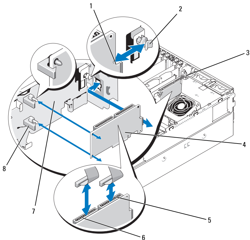
图 3-23. 安装 RAC 卡
