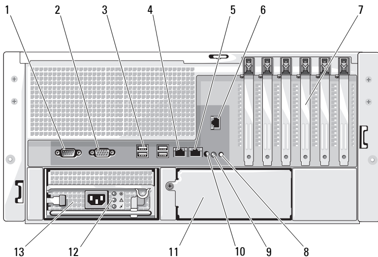
图 1-4. 背面板部件和指示灯
