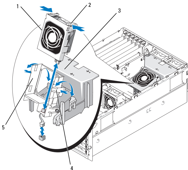
图 3-13. 卸下和更换冷却导流罩风扇
