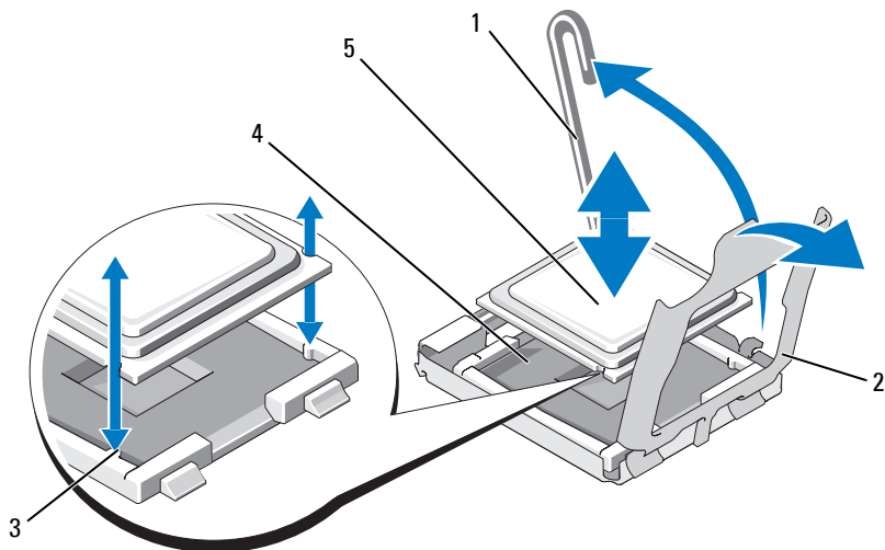
图 3-25. 安装和卸下处理器
