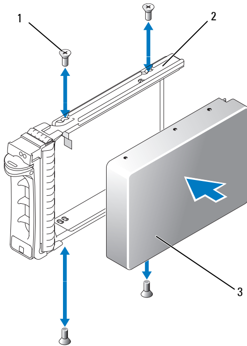
图 3-8. 将 SATA 硬盘驱动器安装到 SATA 驱动器托盘中
