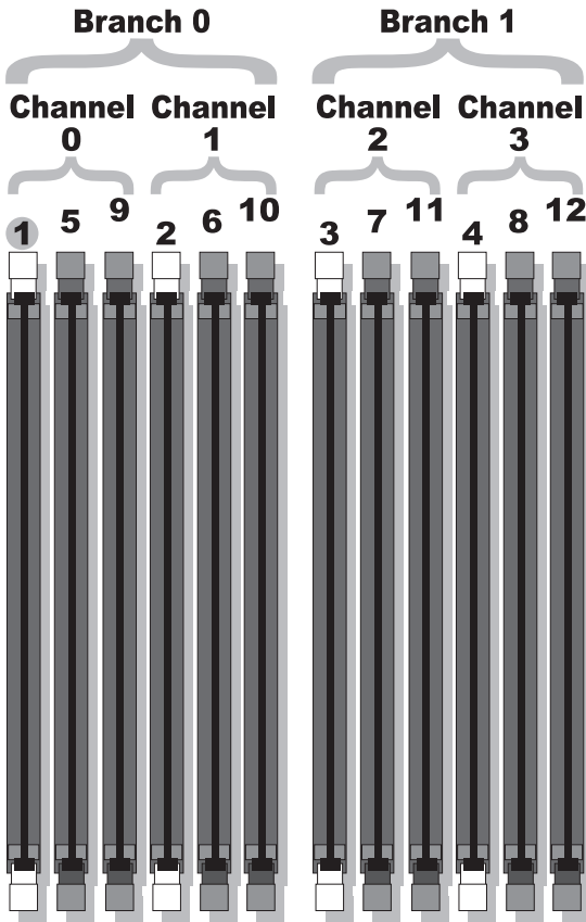
图 3-21. DIMM 插槽
