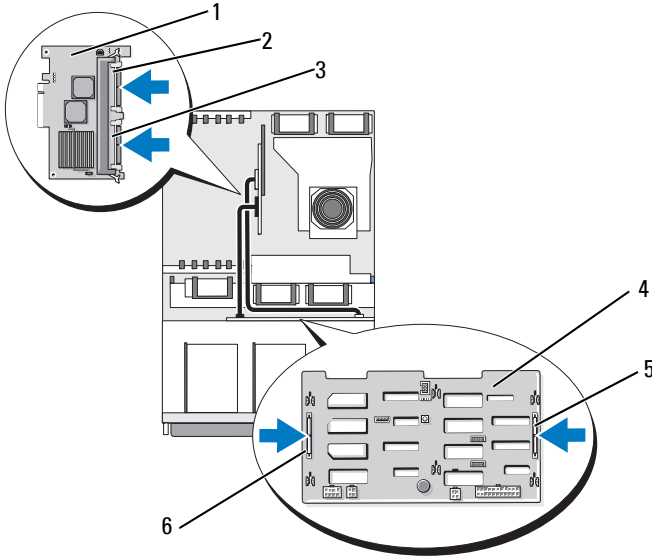
图 3-30. 将 SAS RAID 控制器连接至 1x8 背板
