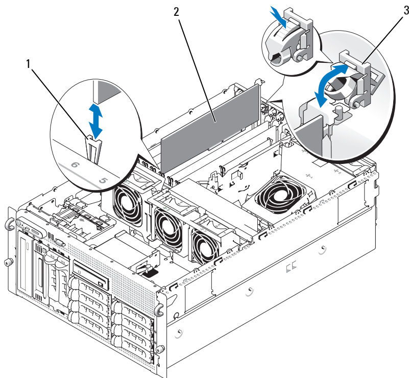
图 3-15. 安装和卸下扩充卡
