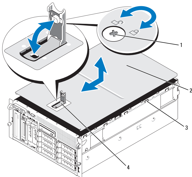
图 3-4. 安装和卸下主机盖
