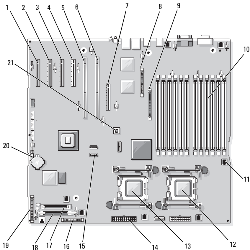
图 6-2. 系统板连接器
