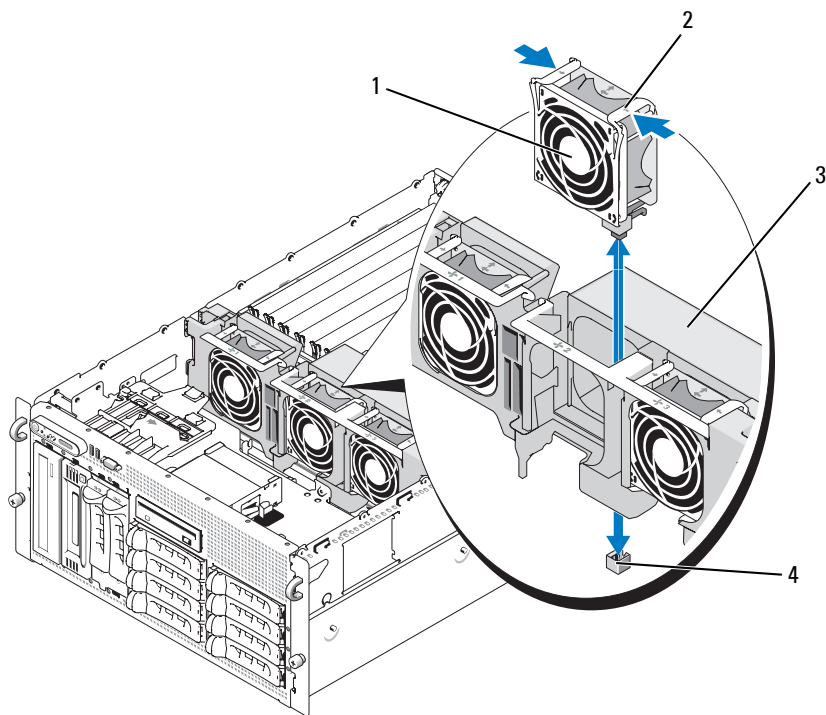
图 3-12. 将风扇安装到风扇支架中和从风扇支架中卸下风扇
