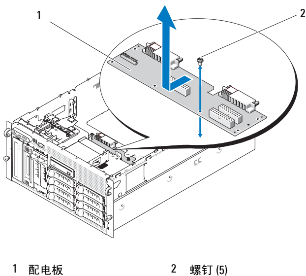
图 3-34. 卸下配电板
