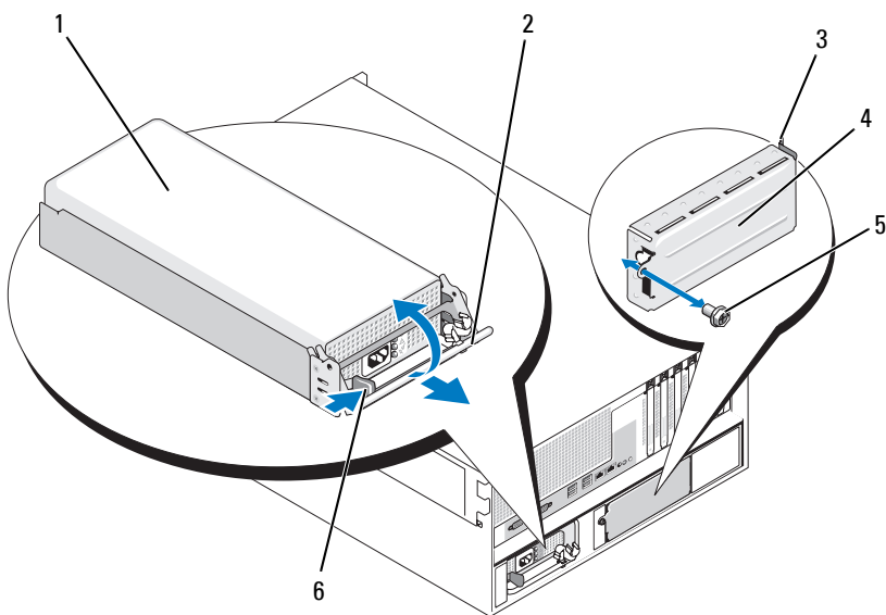
图 3-10. 安装和卸下电源设备
