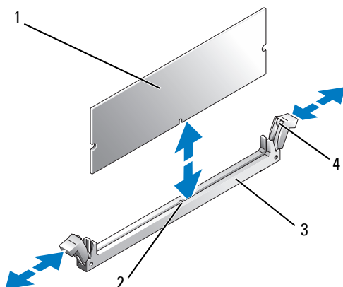
图 3-22. 安装和卸下内存模块
